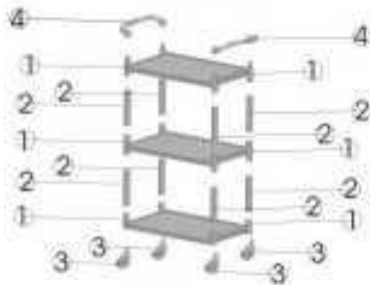
Чертеж сборки
